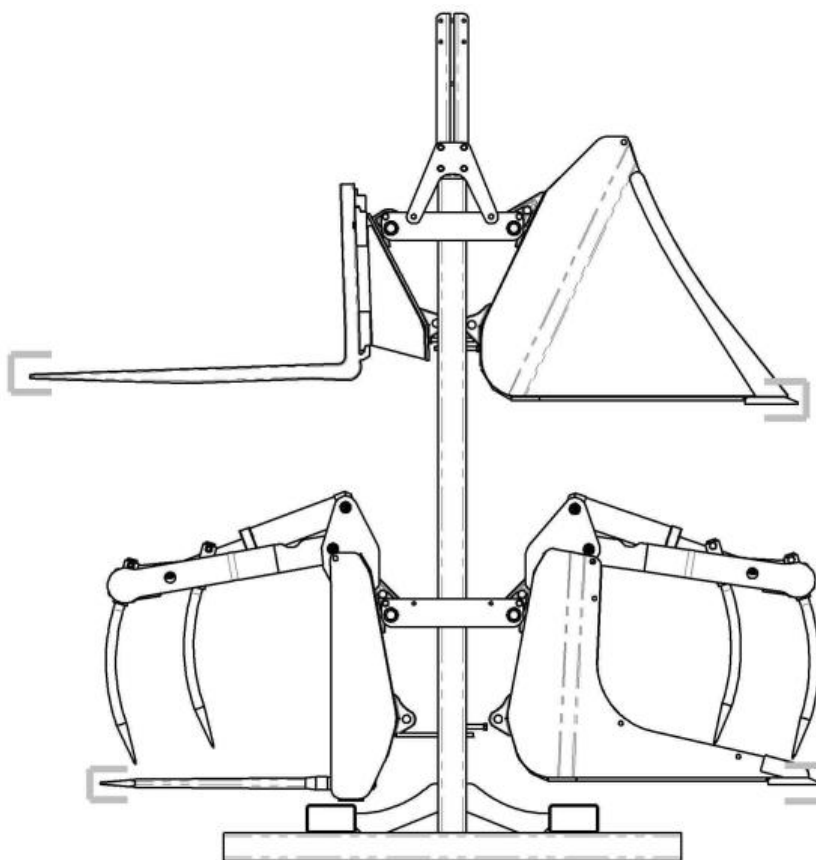
Illustration 3 - Support d'outils équipé des outils de chargeur frontal
