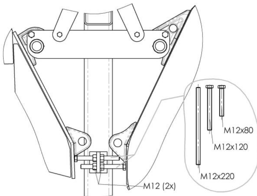
Illustration 4 - Réglage de l'inclinaison d'outil au moyen d'une butée vissée
