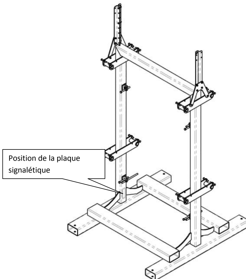
Illustration 2 - Support d'outils monté sans outil de chargeur frontal
