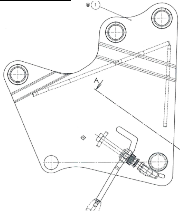
vorgesetzte Säule
