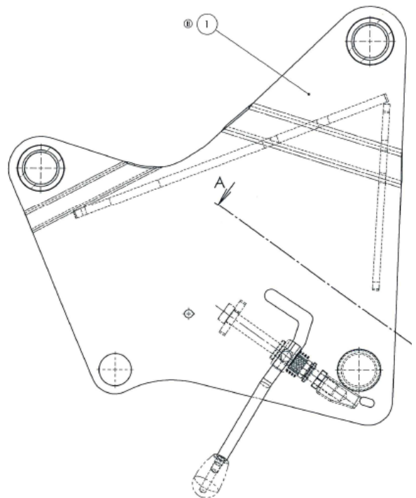
vorgesetzte Säule
